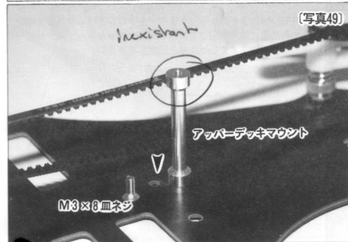
〔写真49〕 No.5 の袋からアッパーデッキマウントとM3 x 8 mm 皿ネジを取り出し、矢印の穴に取り付けます。
