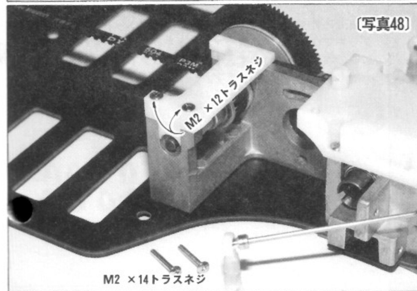
〔写真48〕 モーターマウントキャップはM2 x 12mm、M2 x 14mm トラスネジを使用します。後ろから見て左側はM2 x 12mm トラスネジを使用します。右側はまだつけないで下さい。
