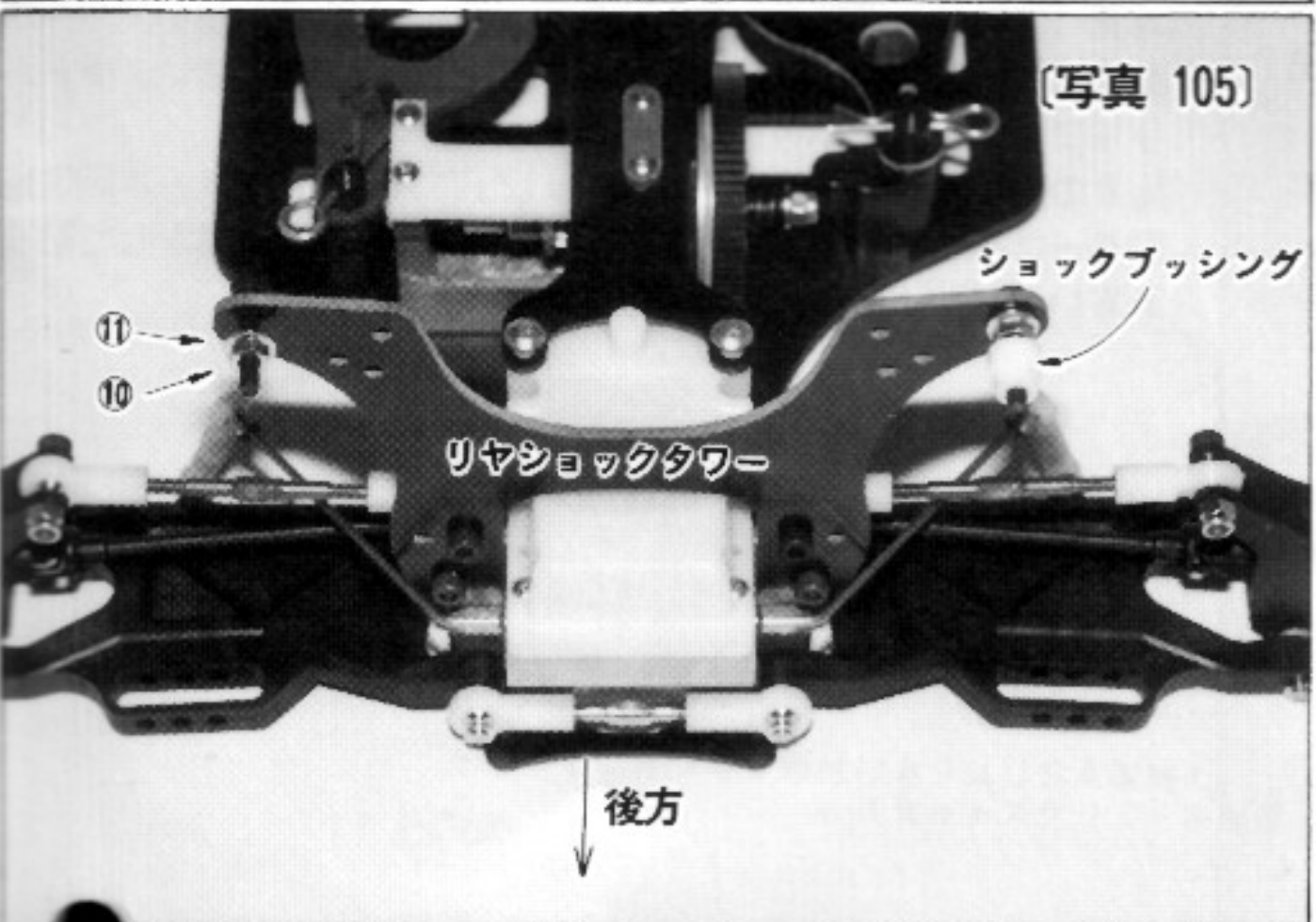
[写真 105] それではリヤショックの取付けにかかります。M3×13mmキャップスクリューをリヤショックタワー前方より差込みM3フランジナットでガッチリ固定して下さい。写真の右のようにショックブッシングを入れます。
