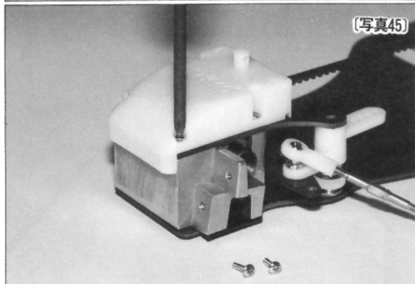
M2×8トラスネジ
