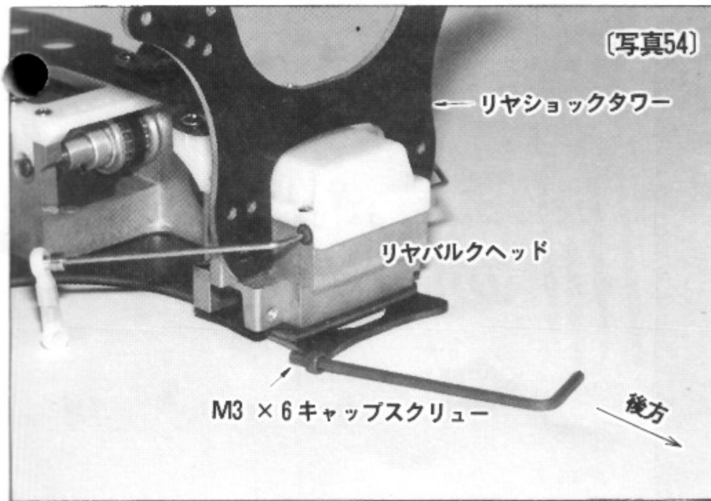
[写真54] リヤショックタワーはリヤバルクヘッドの取付け部のところに後側から立てかけて、フロント同様にM3×6mmキャップスクリューを2本使用してリヤバルクヘッドにしっかりと固定して下さい。
