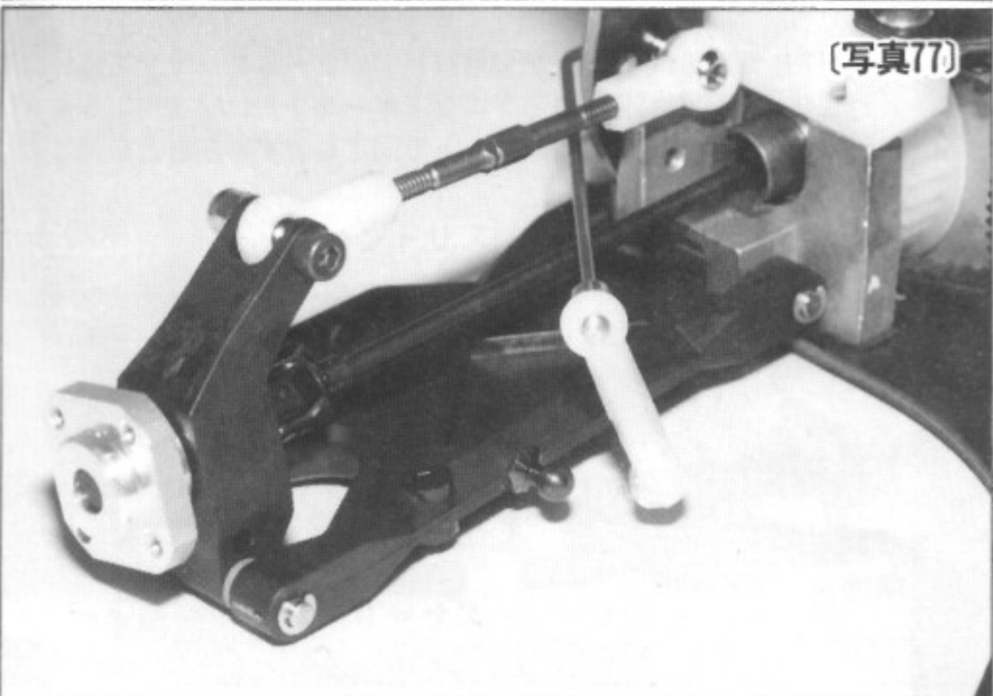
[写真77] リヤアンチロールバーにつけたボールエンドキャップをリヤサスアームのロッドエンドスチールボールに入れます。
