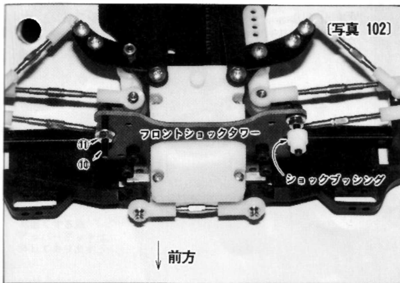
[写真 102] さあ、それではフロントショックの取付けにかかります。M3×18mmキャップスクリューをフロントショックタワー後方より差込み、M3フランジナットでガッチリ固定して下さい。写真の右のようにショックブッシングを入れます。
