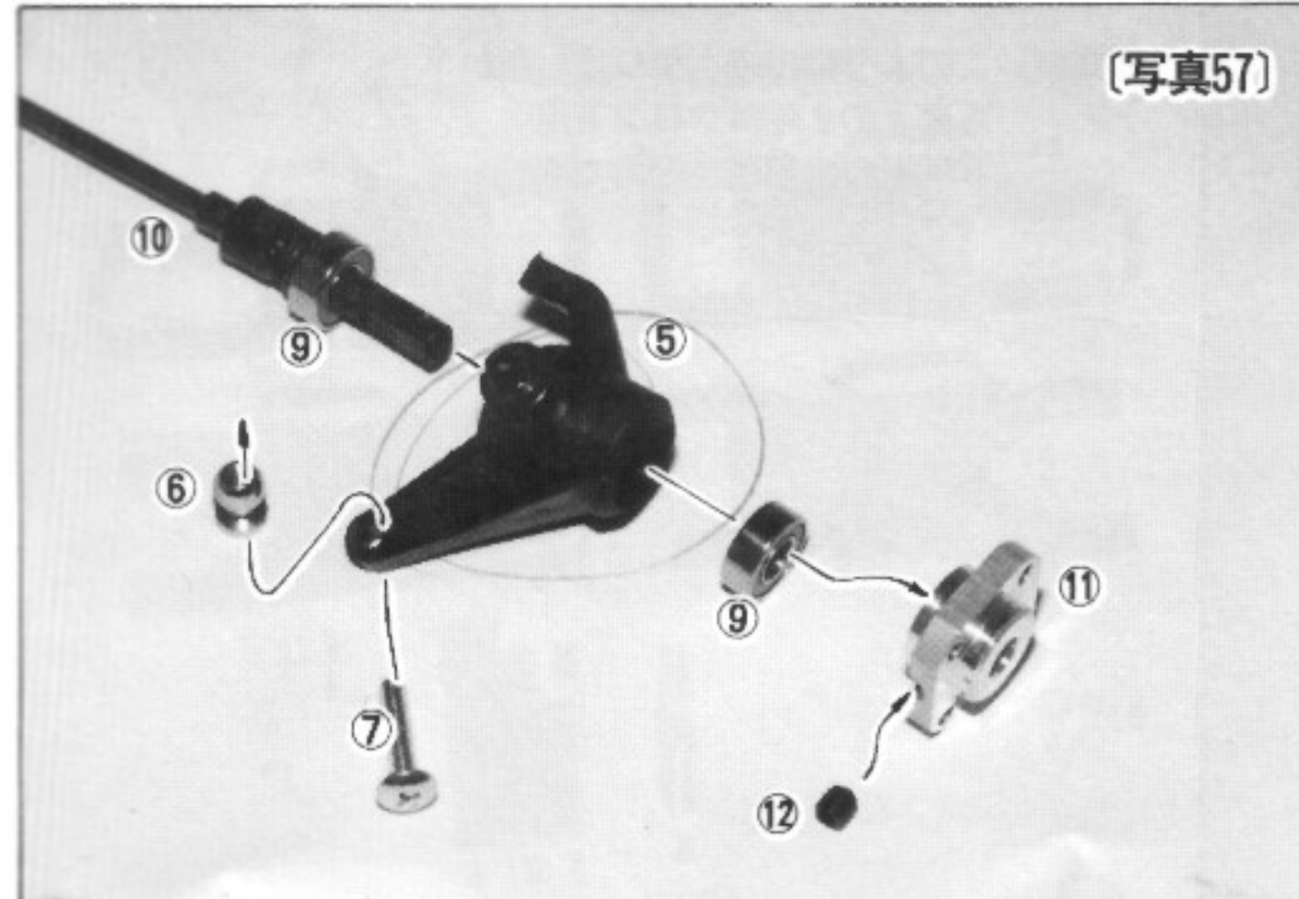
[写真57] フロントドライブシャフト部分の組立にはいります。組立は簡単です。写真の矢印の並び順に組んで、ホイールハブを取付ける時に、ドライブシャフトのDカット面を合わせてセットスクリューを締めます。
