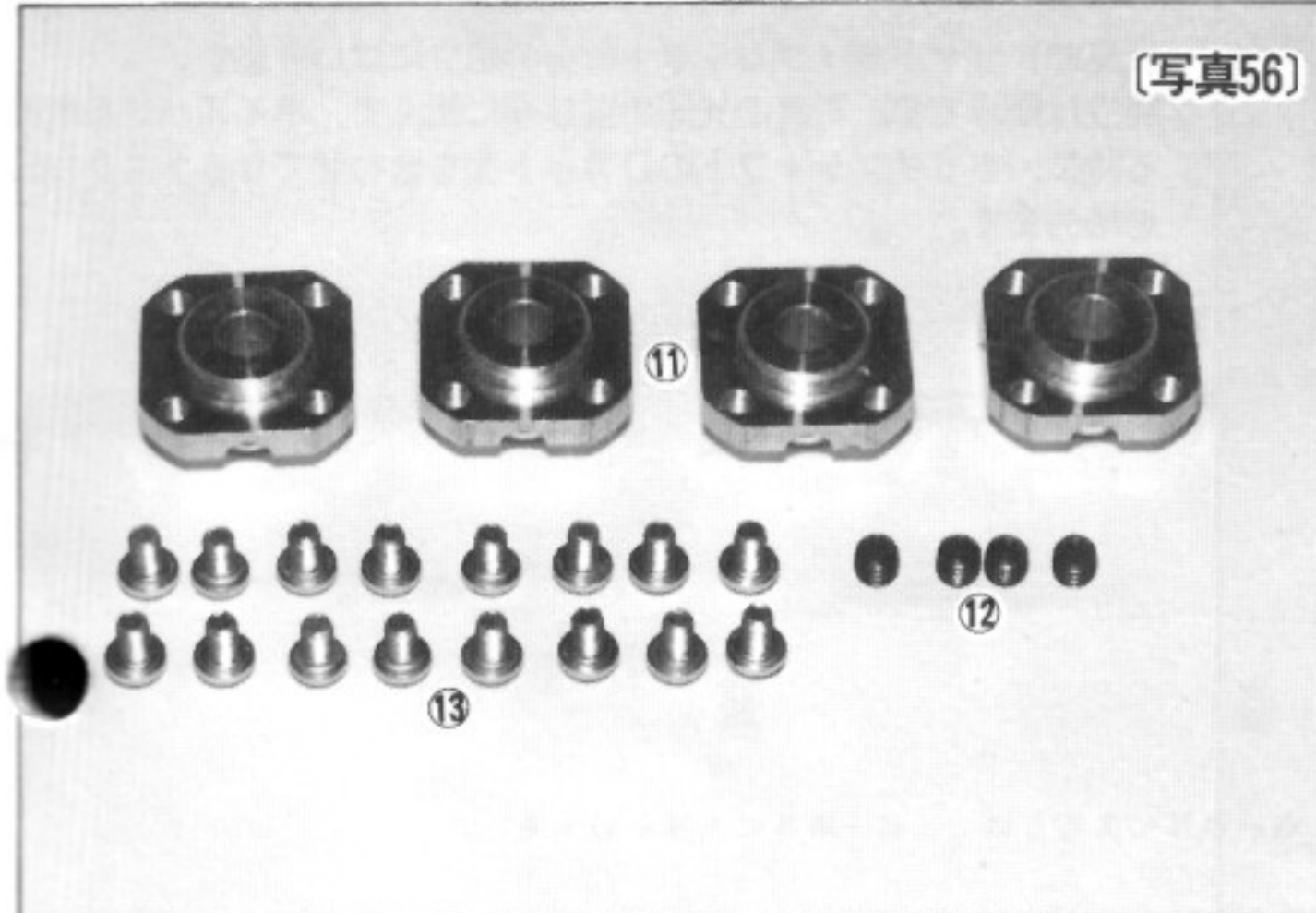
[写真56] No.10のホイールハブの入った袋を取り出して内容を確認して下さい
