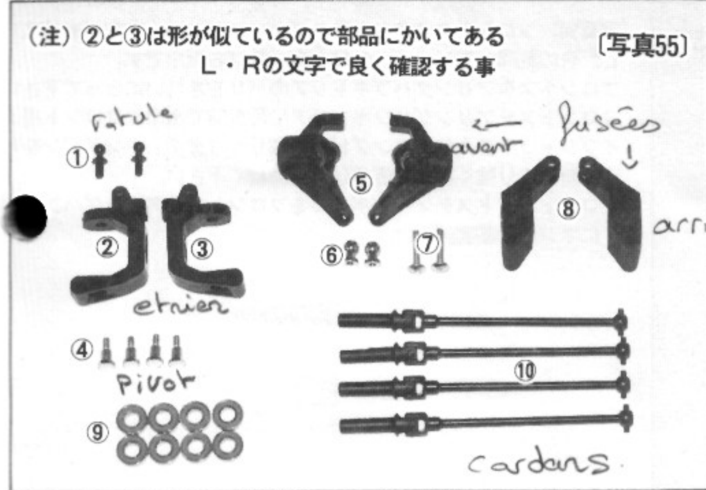
[写真55] No.9のドライブシャフトなどの入った袋を取り出して内容を確認して下さい。
