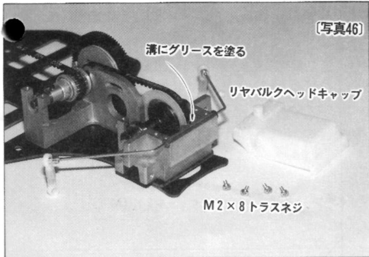
〔写真46〕 リヤバルクヘッドの一番後にある溝に少しシリコングリスを塗って、アンチロールバーをのせます。
