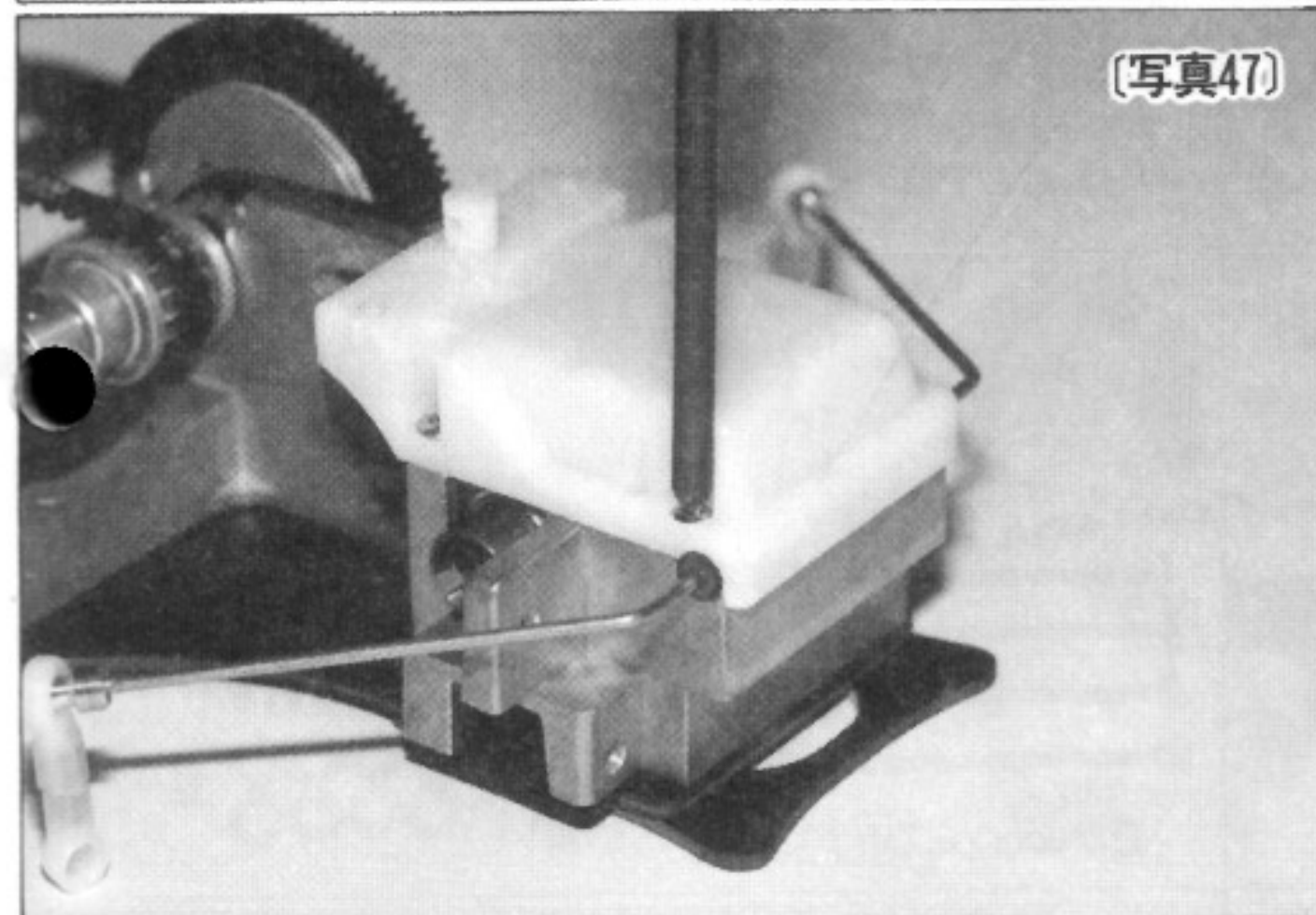
〔写真47〕 リヤバルクヘッドキャップをM2 x 8 トラスネジで取付けます。
