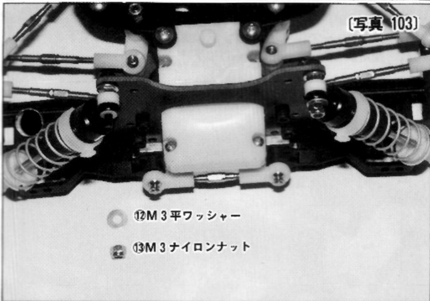
[写真 103] ショックを写真のようにショックブッシングに入れ、M3ワッシャーを入れM3ナイロンナットで固定します。
