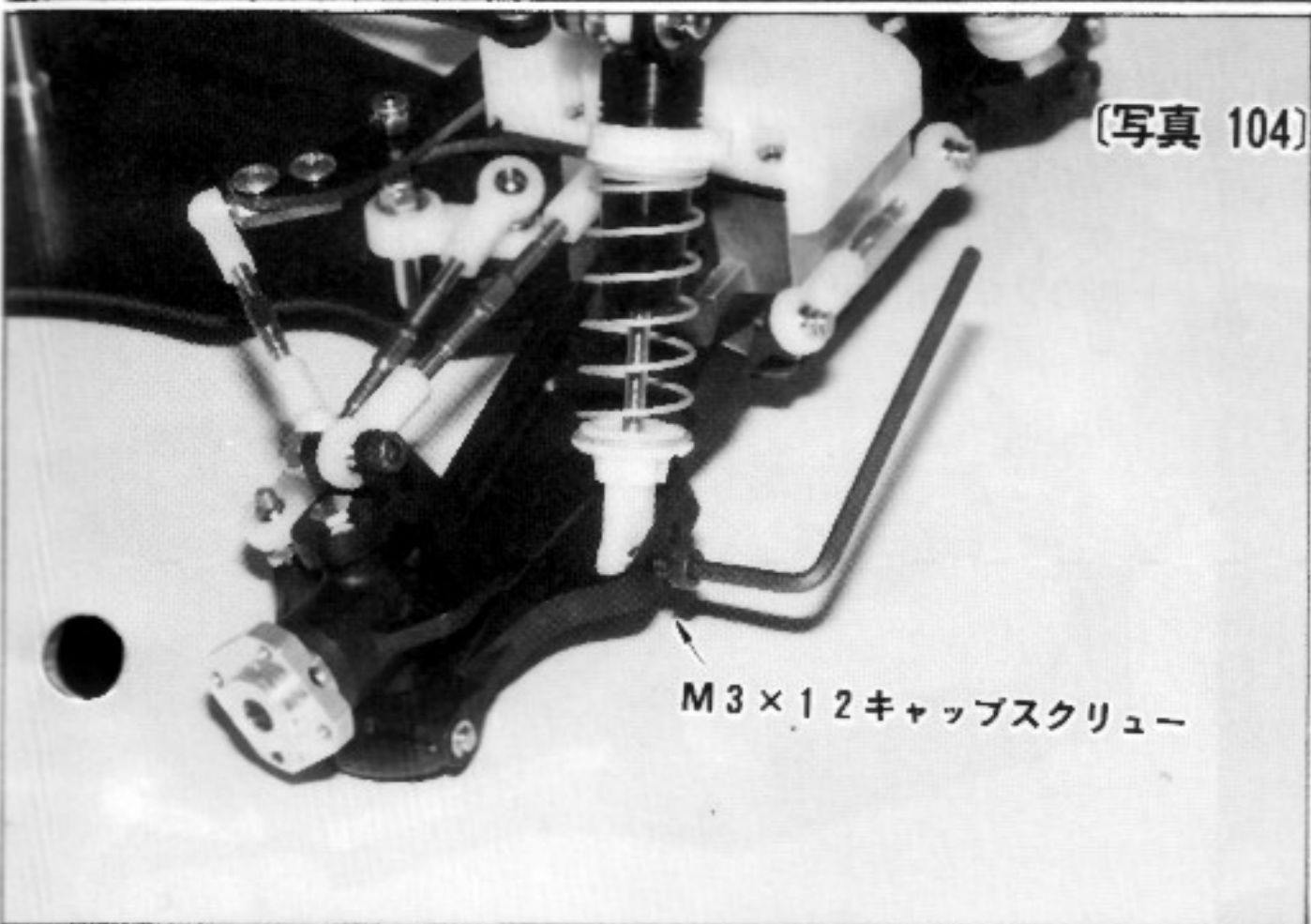
[写真 104] ボールエンドをサスアームに差し込みM3×12mmキャップスクリューで取り付けます。穴位置は外側を使用して下さい。反対側も同様にして取り付けして下さい。
